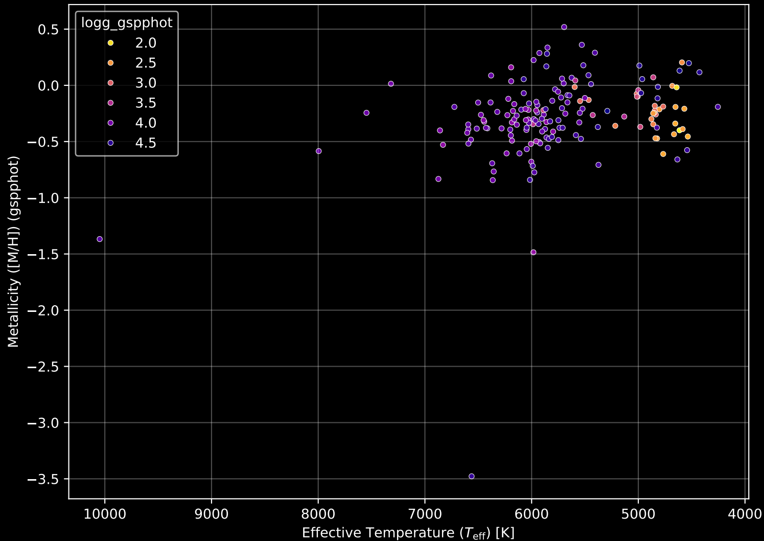
GALAH DR4 Field: [7121] Stellar Population Parameters (n= 168)
